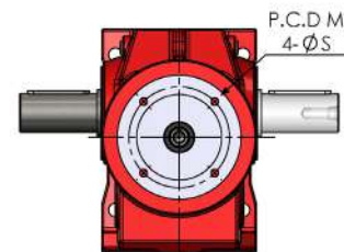
入力孔 Input Bore
