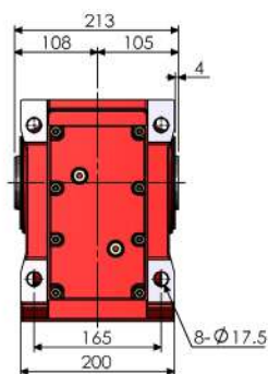
中空出力軸 Output Hollow Shaft
