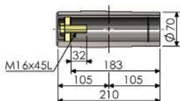
中空出力軸 Output Hollow Shaft
