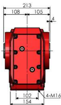
中空出力軸 Output Hollow Shaft
