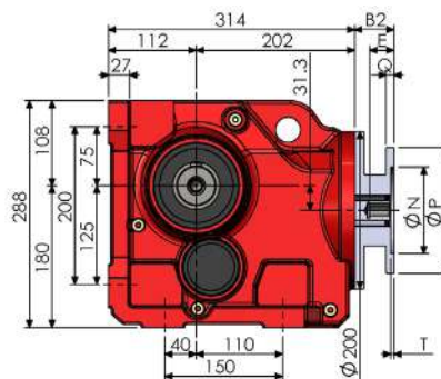
出力軸 Output Shaft
