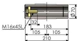
中空出力軸 Output Hollow Shaft
